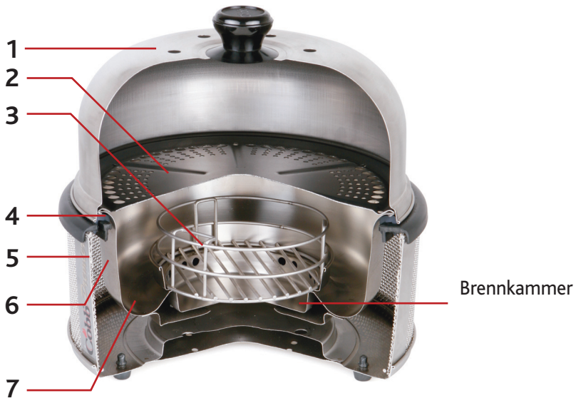
4 Gummiabstandshalter 5 Außenschale
